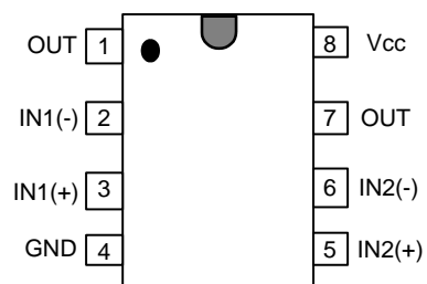
SOP-8 / DIP-8
