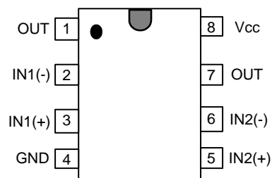
DIP-8
