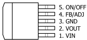
TO-263
