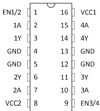
DIP-16
